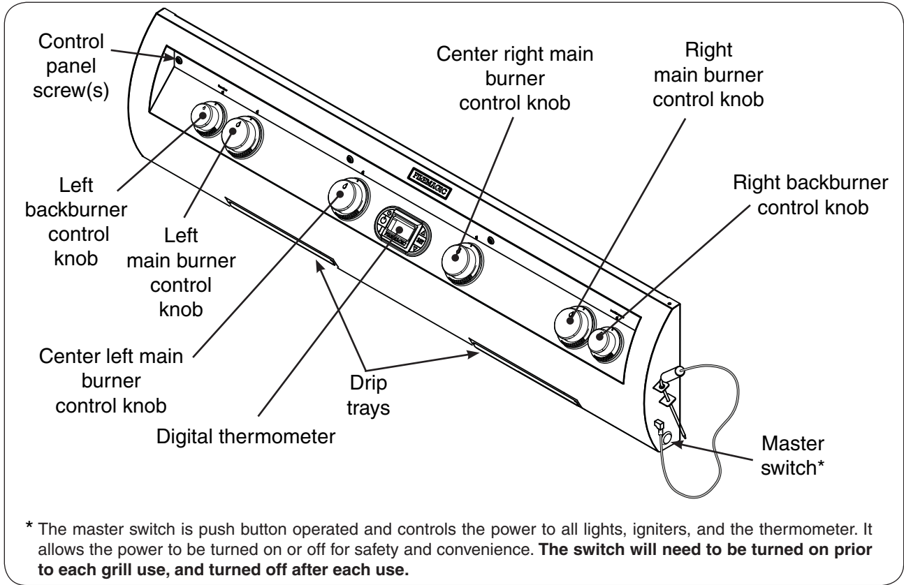
Fig. 22-1 E1060i controls
