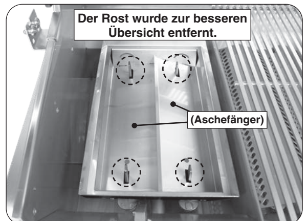
Abb. 33-4 Korbanordnungsdetail
