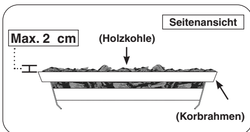
Abb. 34-2 Detail Holzkohle laden
