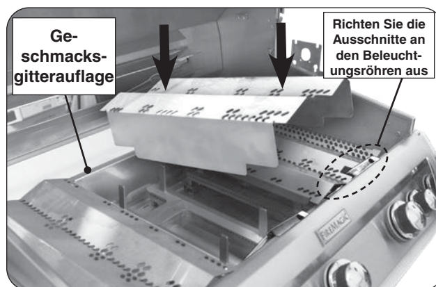
Abb. 23-2 Installieren Sie Aromagitter
