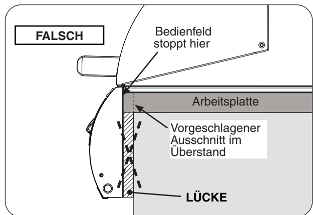
Abb. 22-2 Arbeitsplattenüberstand - falscher Ausschnitt
