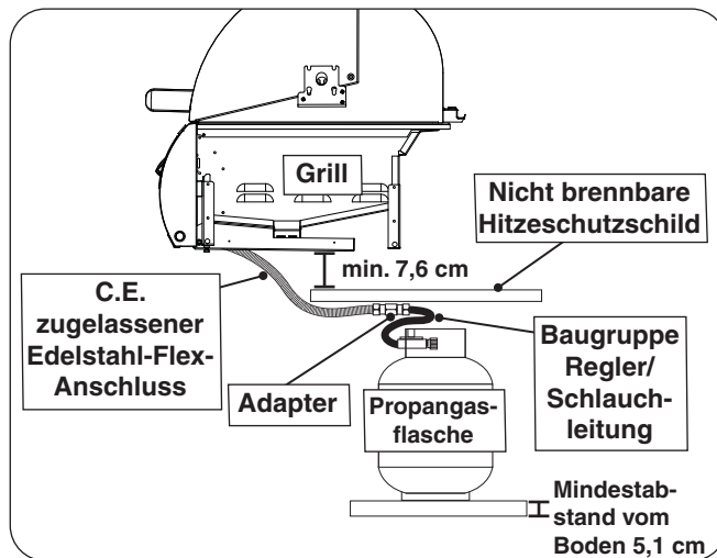
Abb. 8-1 Anordnung Propangasflasche
