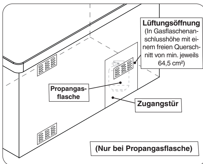
Abb. 8-2 Zusätzliche Lüftungsöffnung für Propangasflasche
