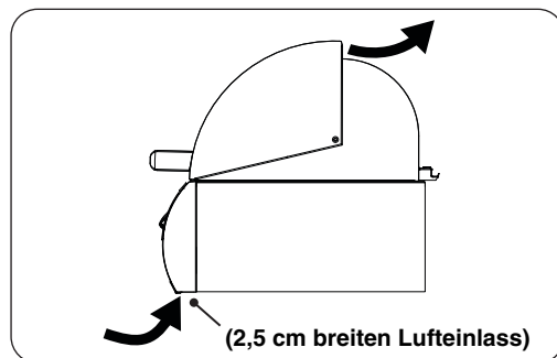
Abb. 11-2 Diagramm Luftstrom
