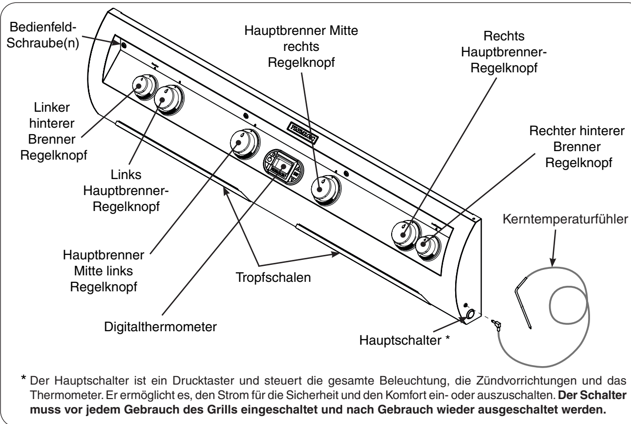
Abb. 26-1 Lage der Steuerung E1060i
