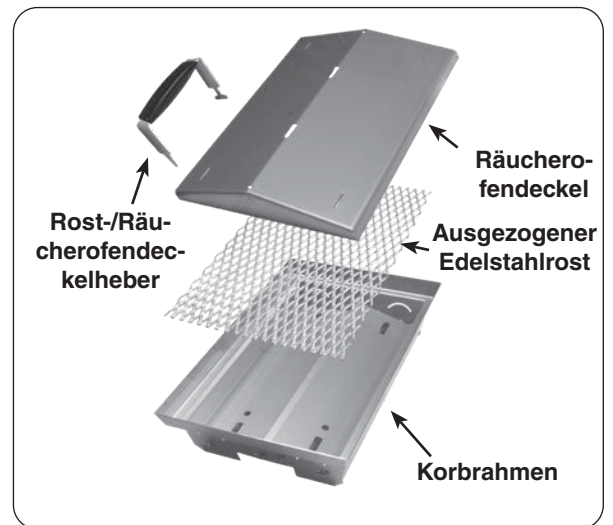
Abb. 33-1 Holzkohle-/Räucherkornteile
