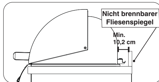
Abb. 10-4 Freiraum bei Fliesenspiegel
