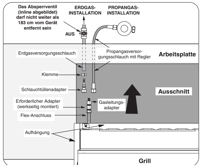
Abb. 22-3 Propangas- und Erdgasdiagramm
