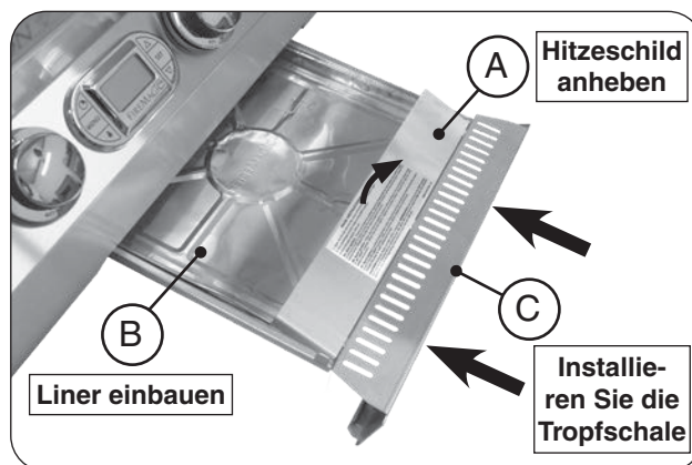
Abb. 24-1 Die Tropfschale montieren
