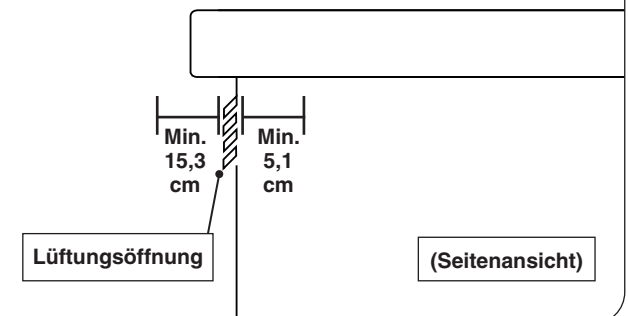
Abb. 7-2 Freiraum Lüftungsöffnung
