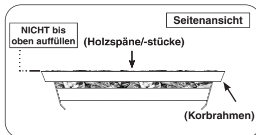
Abb. 34-4 Detail Holzspäne/-stücke laden
