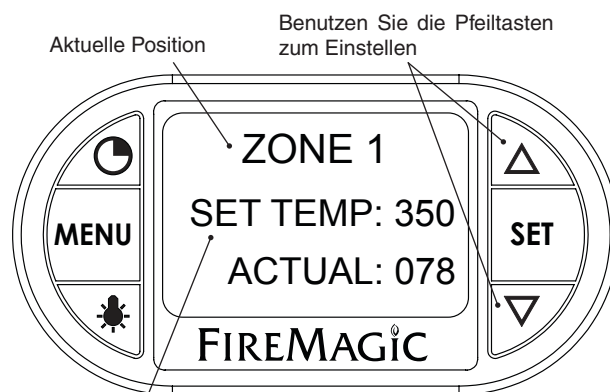
Abb. 30-1 Bildschirm Zonentemperatur (Zone 1 abgebildet)
