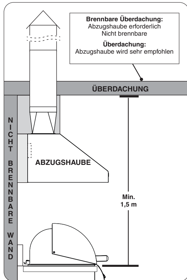
Abb. 9-1 Anforderungen an die Überdachung
