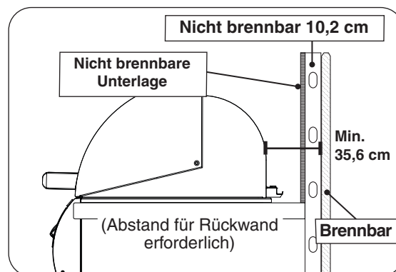
Abb. 10-2 Freiraum 'B' Diagramm
